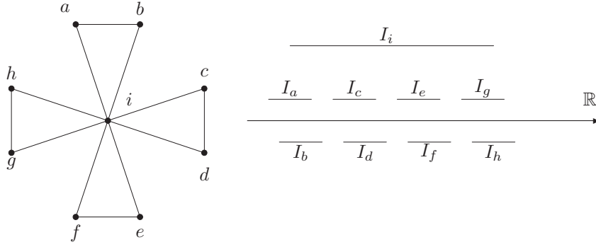
Σχήμα 2.5: Ένα Γράφημα Διαστημάτων (Interval Graph).
