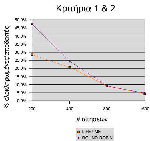
Σχήμα 5.1 Πρώτη Κατηγορία Μετρήσεων. C \in (1, \frac{clientLifetime}{40})
