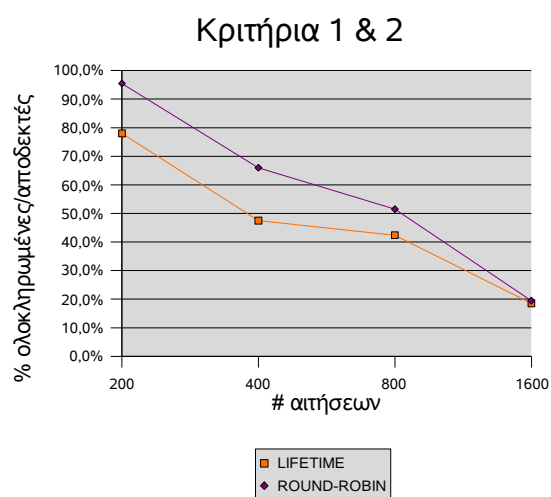
Σχήμα 5.2 Δεύτερη Κατηγορία Μετρήσεων. C \in (1, \frac{clientLifetime}{160})
