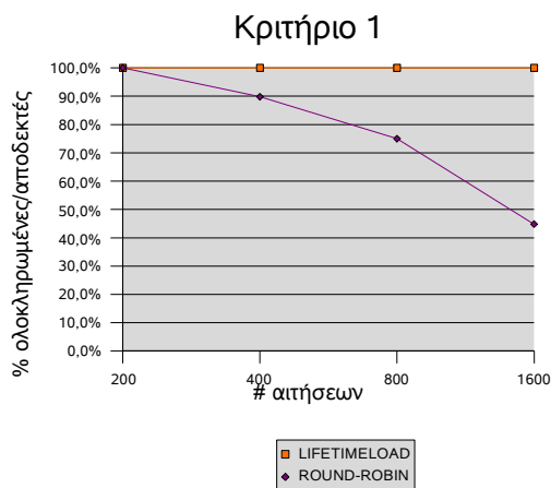
Σχήμα 5.8 Τρίτη Κατηγορία Μετρήσεων. C \in (1, \frac{clientLifetime}{320})
