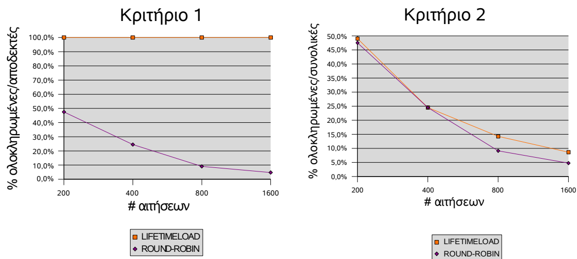
Σχήμα 5.6 Πρώτη Κατηγορία Μετρήσεων. C \in (1, \frac{clientLifetime}{40})
