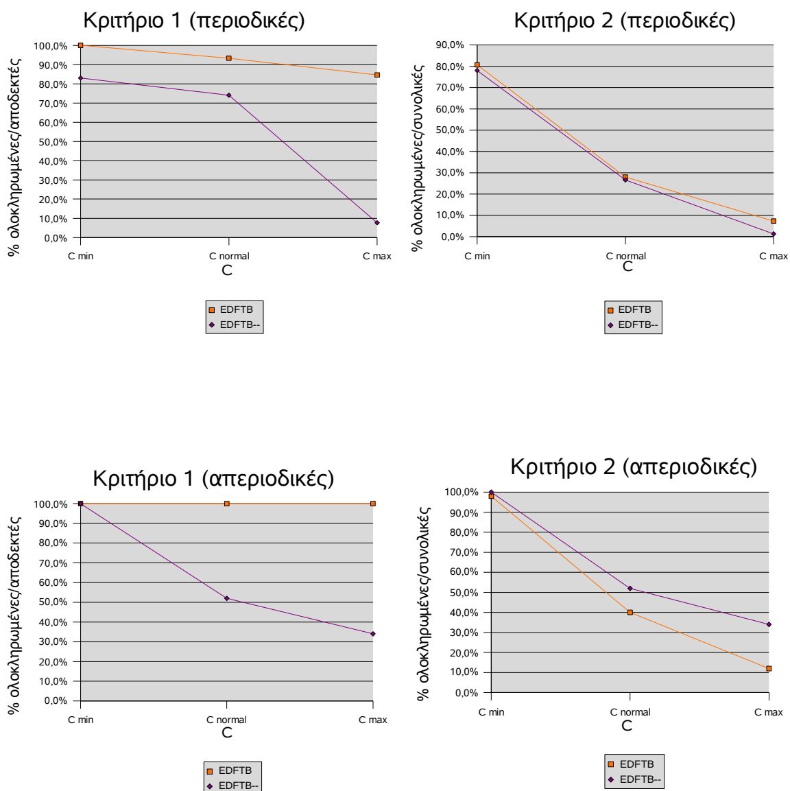
Σχήμα 6.6 Πρώτη Κατηγορία Μετρήσεων.
