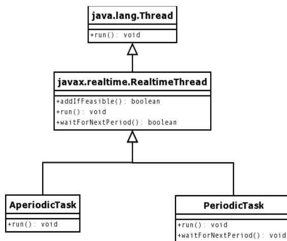
Σχήμα 6.3 Ιεραρχία Κλάσεων PeriodicTask και AperiodicTask .
