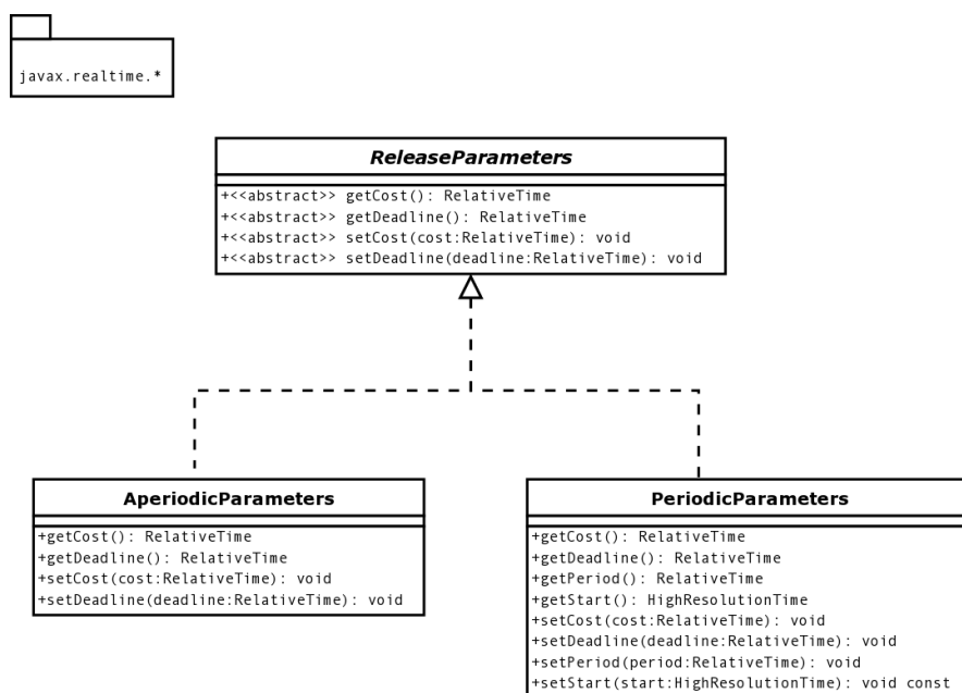
Σχήμα 6.1 Υποκλάσεις της ReleaseParameters .
