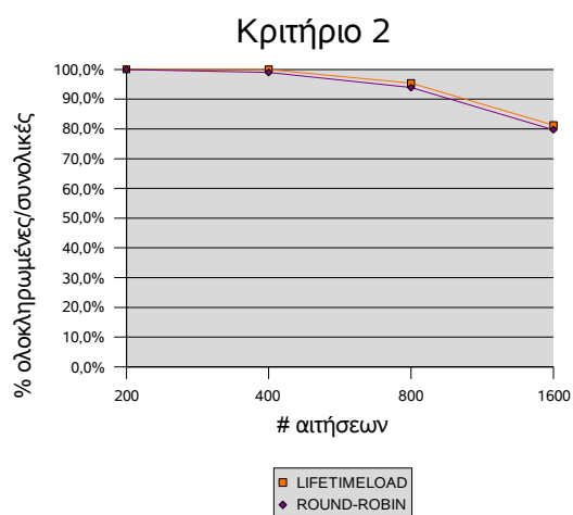
Σχήμα 5.9 Τέταρτη Κατηγορία Μετρήσεων. C \in (1, \frac{clientLifetime}{640})
