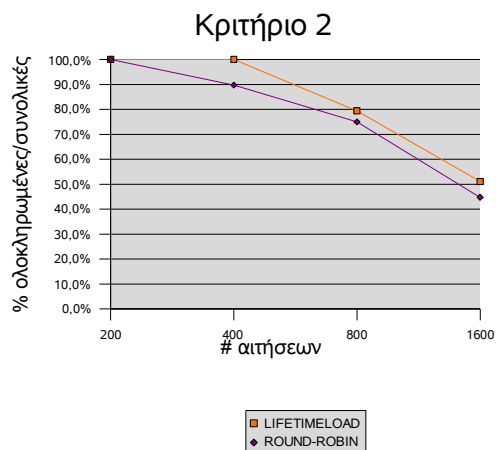
Σχήμα 5.8 Τρίτη Κατηγορία Μετρήσεων. C \in (1, \frac{clientLifetime}{320})
