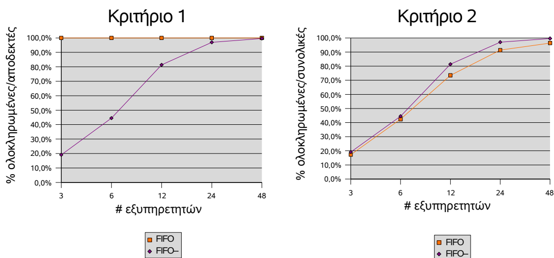
Σχήμα 5.15 Σύγκριση με Αυξανόμενο Αριθμό Εξυπηρετητών.
