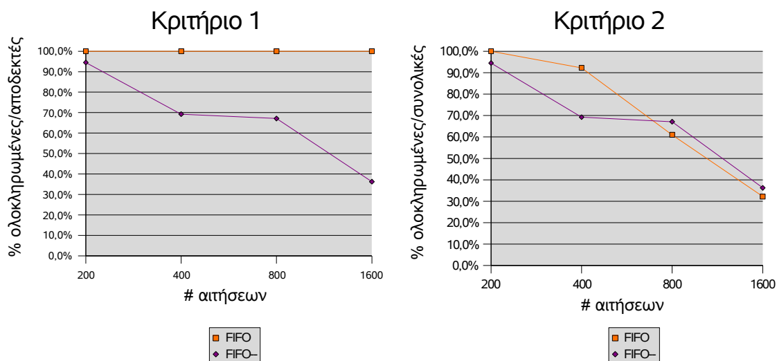
Σχήμα 5.12 Δεύτερη Κατηγορία Μετρήσεων. C \in (1, \frac{clientLifetime}{160})
