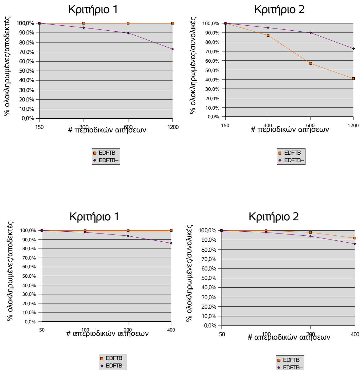
Σχήμα 5.19 Τέταρτη Κατηγορία Μετρήσεων. C \in (1, \frac{clientLifetime}{640})
