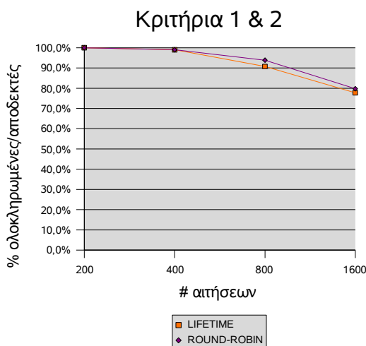
Σχήμα 5.4 Τέταρτη Κατηγορία Μετρήσεων. C \in (1, \frac{clientLifetime}{640})
