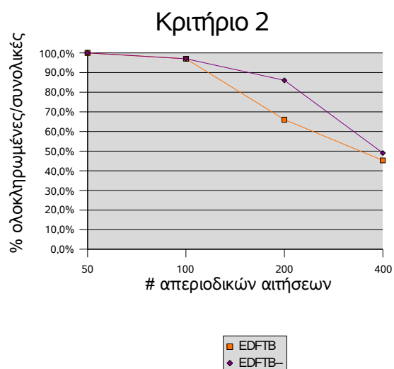
Σχήμα 5.17 Δεύτερη Κατηγορία Μετρήσεων. C \in (1, \frac{clientLifetime}{160})
