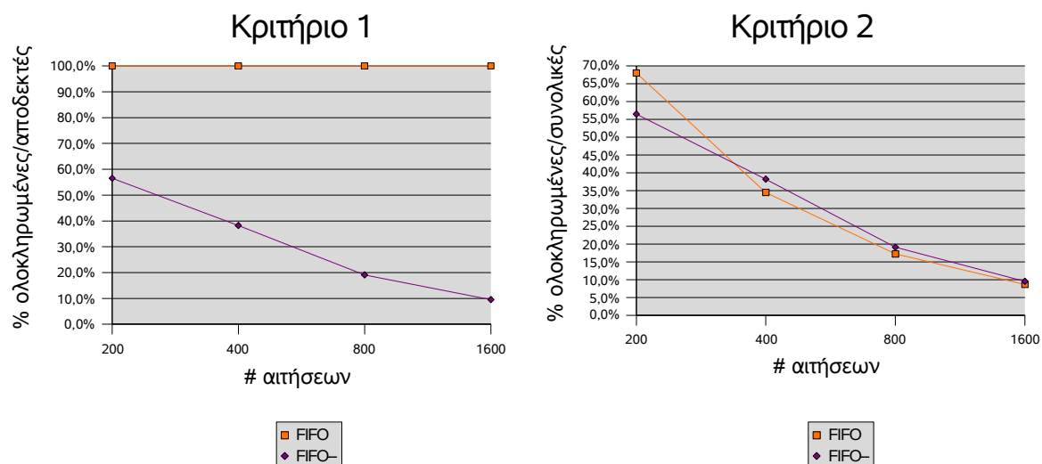
Σχήμα 5.11 Πρώτη Κατηγορία Μετρήσεων. C \in (1, \frac{clientLifetime}{40})
