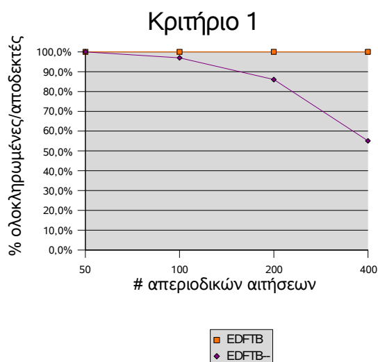
Σχήμα 5.17 Δεύτερη Κατηγορία Μετρήσεων. C \in (1, \frac{clientLifetime}{160})
