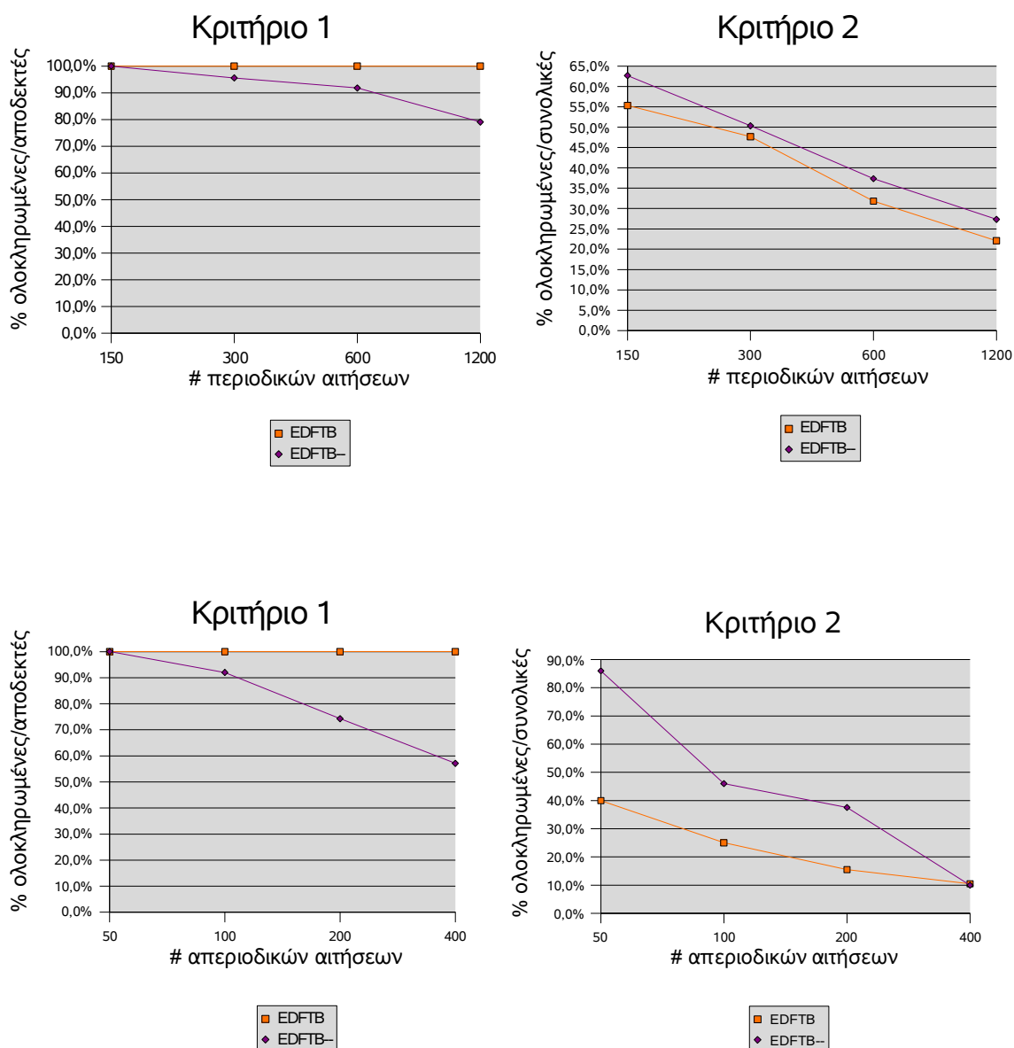
Σχήμα 5.16 Πρώτη Κατηγορία Μετρήσεων. C \in (1, \frac{clientLifetime}{40})
