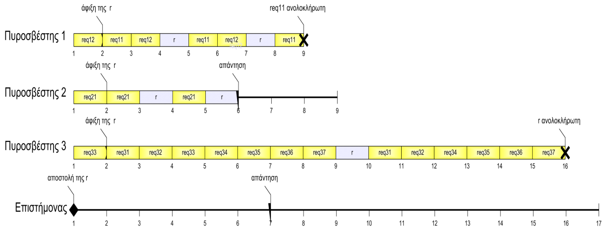
Σχήμα 4.2 Εφαρμογή της Πολιτικής LifetimeLoad.
