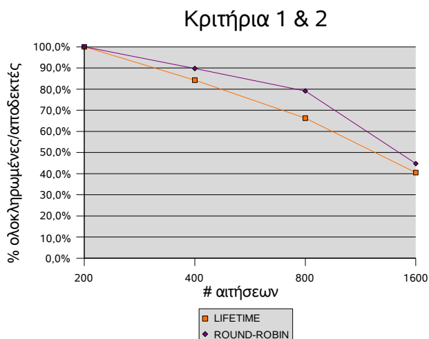
Σχήμα 5.3 Τρίτη Κατηγορία Μετρήσεων. C \in (1, \frac{clientLifetime}{320})
