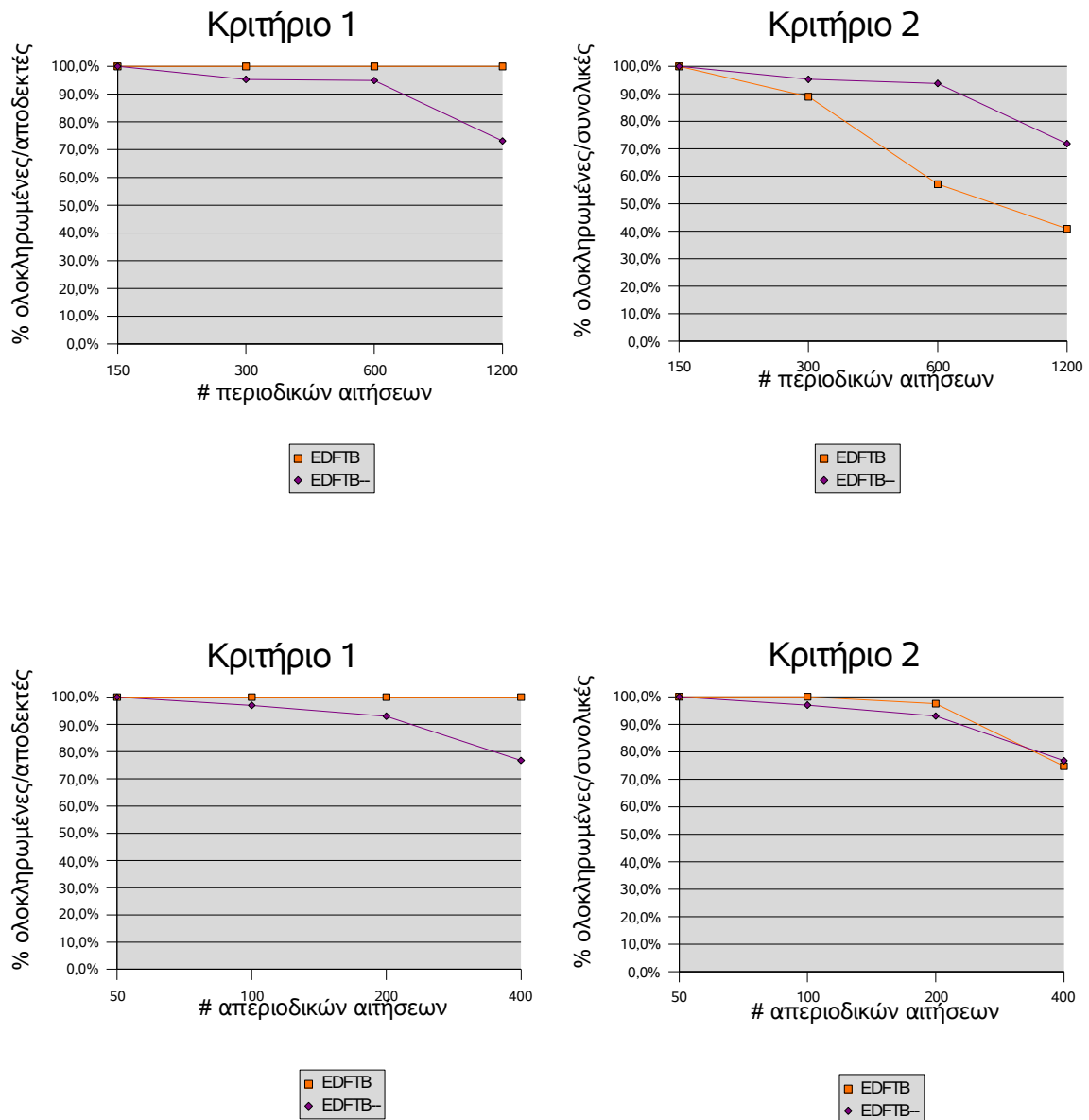
Σχήμα 5.18 Τρίτη Κατηγορία Μετρήσεων. C \in (1, \frac{clientLifetime}{320})
