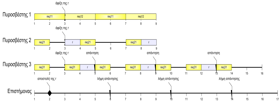
Σχήμα 4.5 Εφαρμογή της Πολιτικής EDFTB για Περιοδικές Αιτήσεις.
