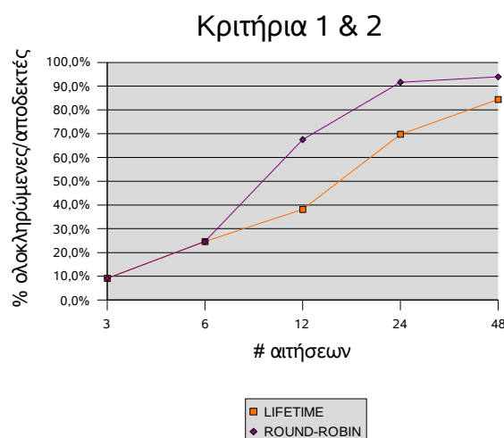
Σχήμα 5.5 Σύγκριση με Αυξανόμενο Αριθμό Εξυπηρετητών.
