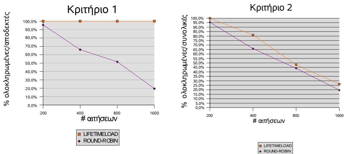
Σχήμα 5.7 Δεύτερη Κατηγορία Μετρήσεων. C \in (1, \frac{clientLifetime}{160})
