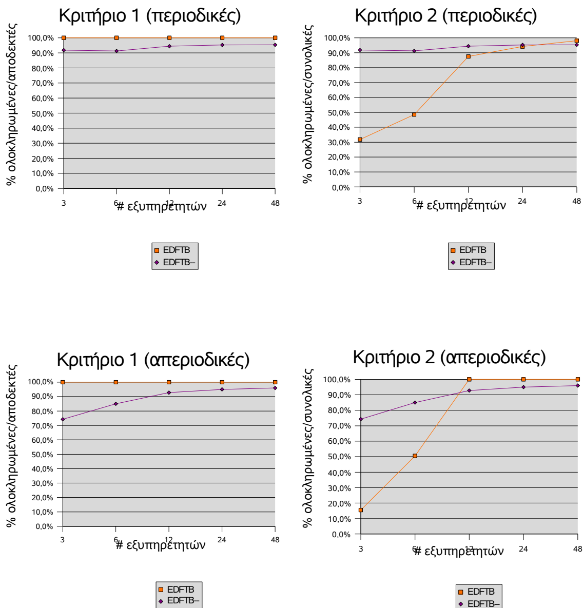
Σχήμα 5.20 Σύγκριση με Αυξανόμενο Αριθμό Εξυπηρετητών.
