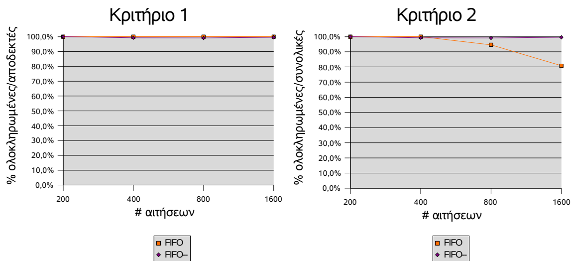
Σχήμα 5.14 Τέταρτη Κατηγορία Μετρήσεων. C \in (1, \frac{clientLifetime}{640})
