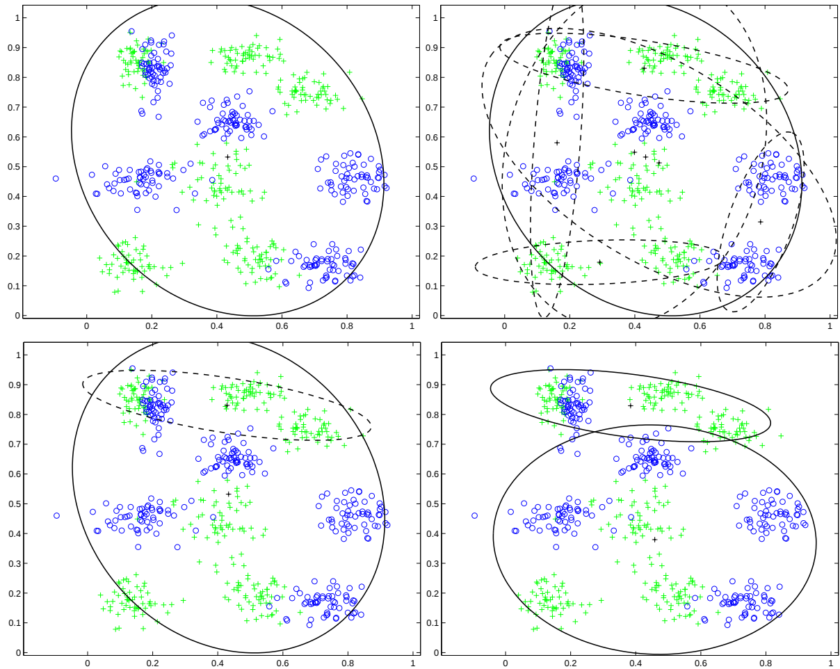
Σχήμα 6.5: Η αυξητική διαδικασία προσθήκης των δύο πρώτων συνιστωσών του δικτύου PRBF. Οι υπάρχουσες συνιστώσες του δικτύου έχουν σχεδιαστεί με συνεχείς γραμμές και οι υποψήφιες συνιστώσες με διακεκομμένες.
