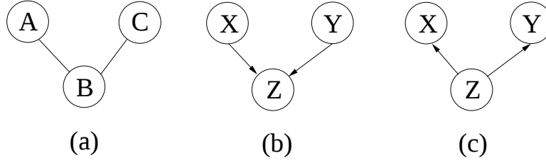
Σχήμα 2.1: Τρία τυπικά γραφικά μοντέλα.
