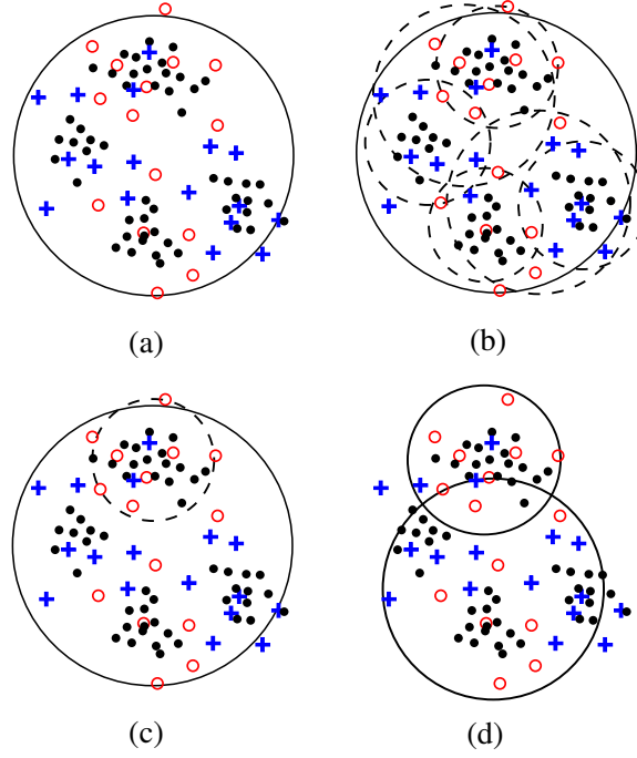
Σχήμα 7.1: Η προσθήκη των δύο πρώτων συνιστωσών. Οι συνιστώσες του δικτύου σχεδιάστηκαν με συνεχείς γραμμές, και οι υποψήφιες συνιστώσες με διακεκομμένες. Οι κουκίδες αναπαριστούν τα ταξινομητά πρότυπα σε ένα πρόβλημα δύο κατηγοριών.
