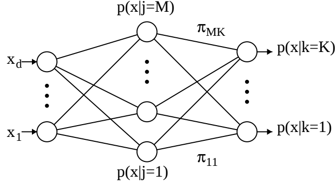
Σχήμα 6.1: Το πιθανοτικό δίκτυο RBF.
