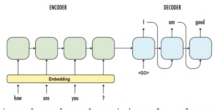
Σχήμα 3.8: Δίκτυο LSTM
