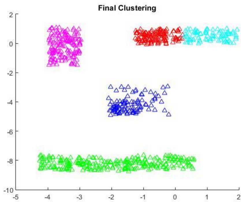
Σχήμα 5.3.23 Dtest Rectangles: Agglodip (All to all, Αρχικό K = 8 )
