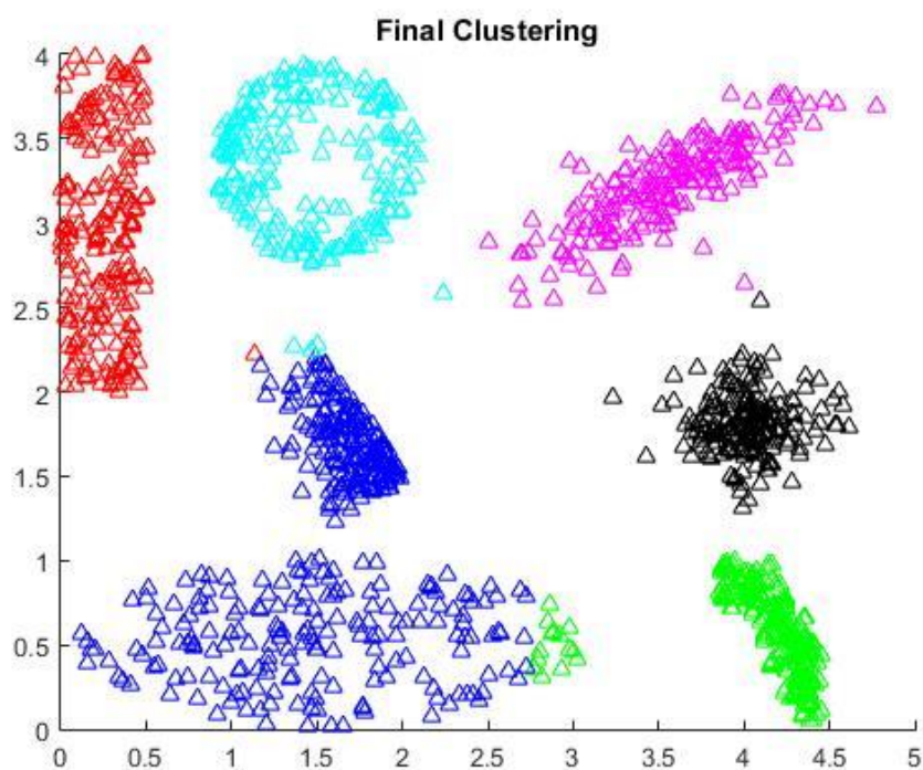
Σχήμα 5.3.11 Combosetting: Agglodip (Graph, Αρχικό K = 21 )
