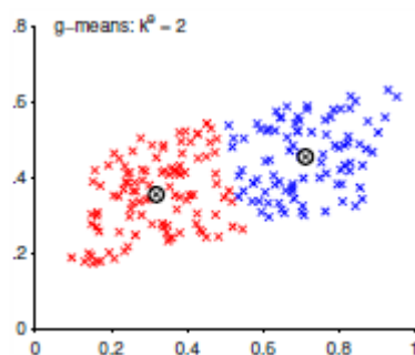
Σχήμα 3.4.6 Ομοιόμορφη G-Means
