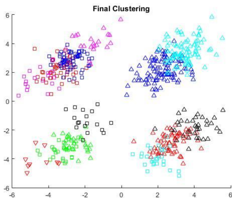
Σχήμα 5.3.1 Kmeansdata: X-Means
