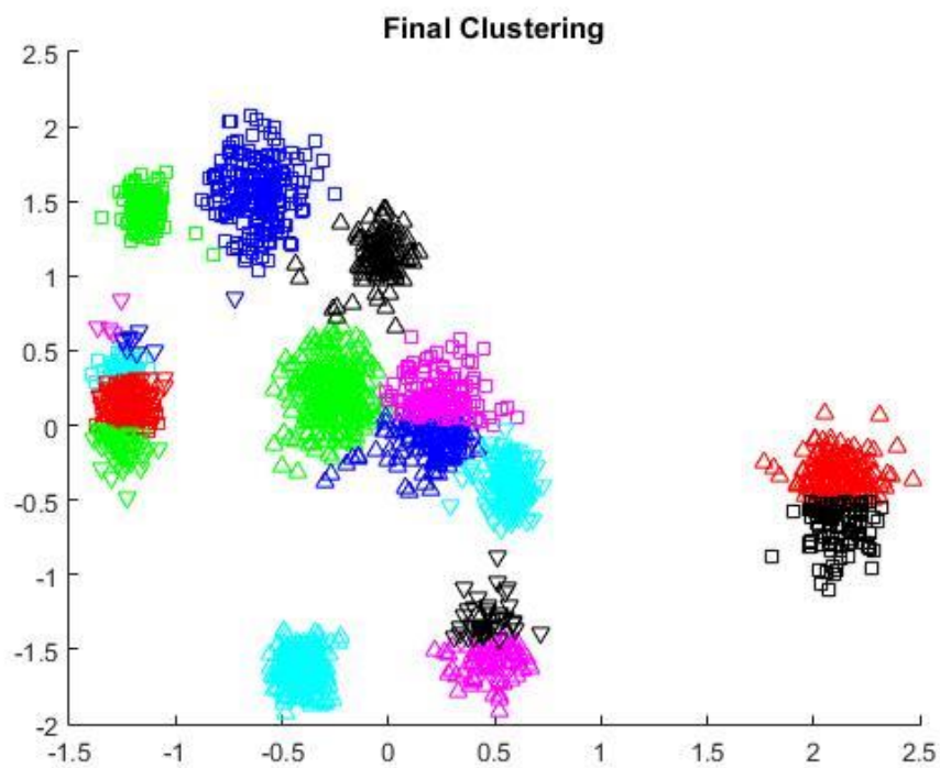
Σχήμα 5.3.26 X10: X-Means
