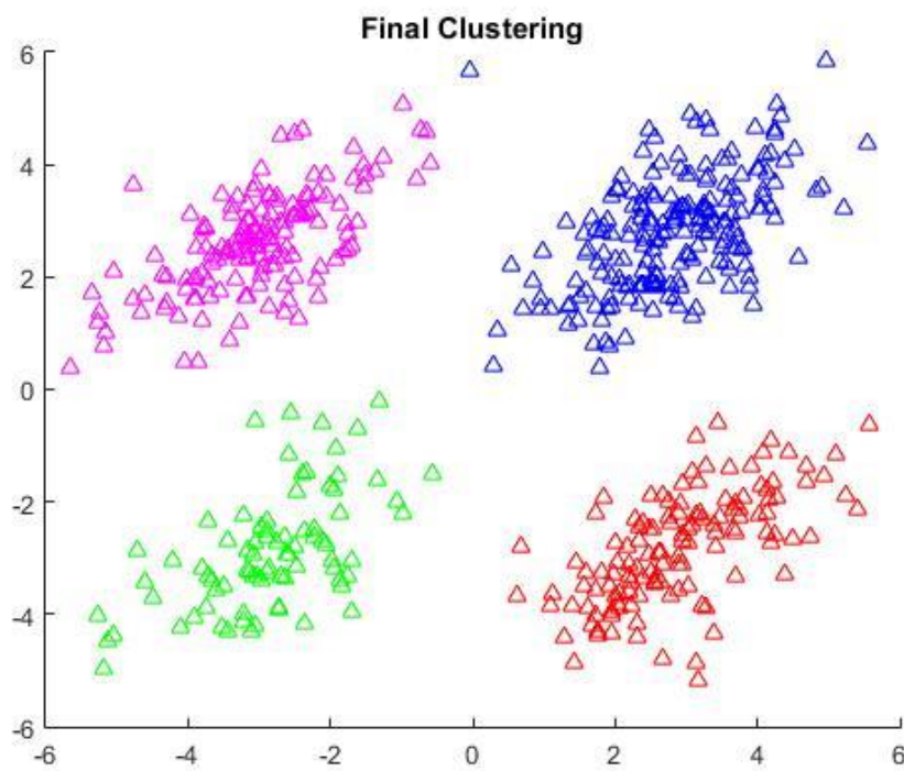
Σχήμα 5.3.2 Kmeansdata: G-Means
