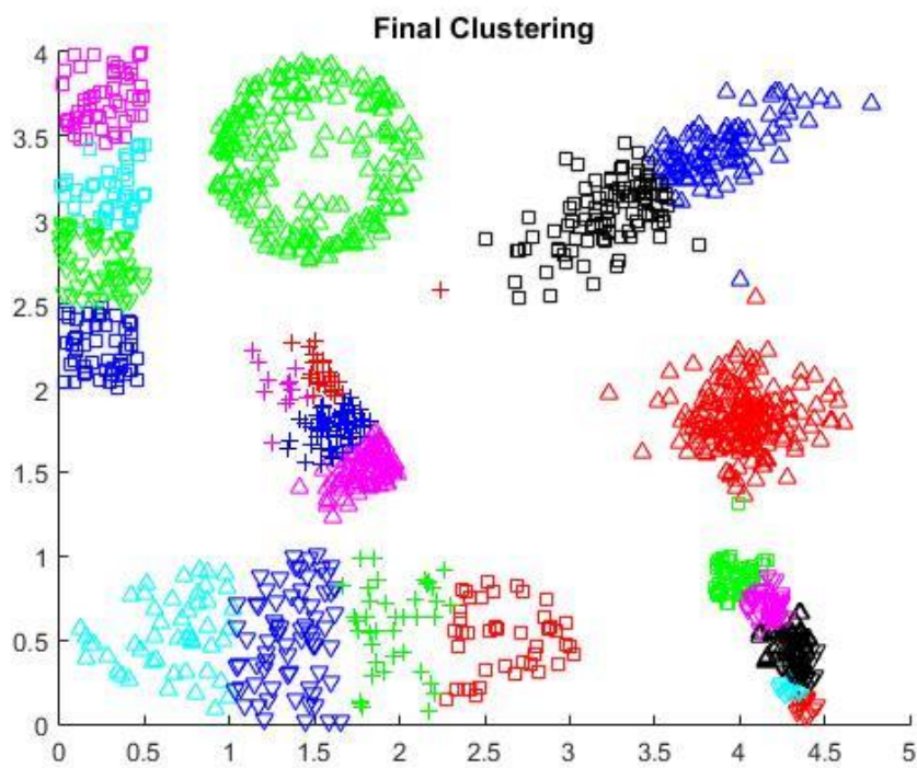
Σχήμα 5.3.4 Combosetting: X-Means
