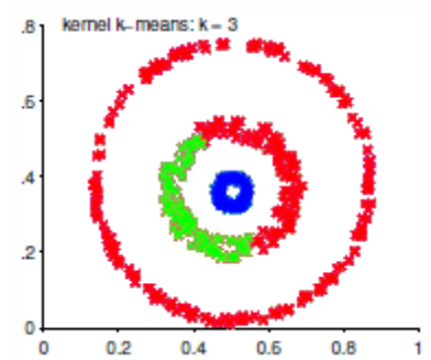
Σχήμα 3.4.11 Kernel K-Means
