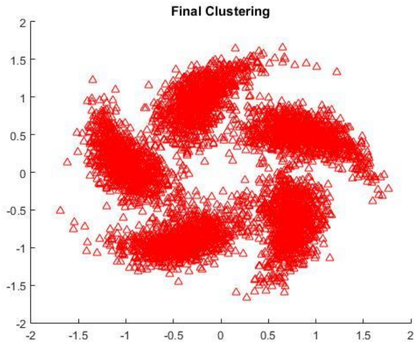
Σχήμα 5.3.12 Pinwheel: X-means
