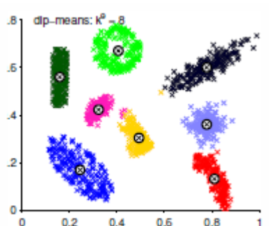
Σχήμα 3.4.7 Μονοτροπικές Dip-Means
