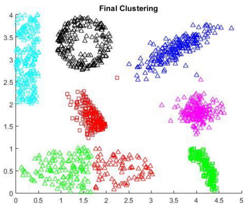
Σχήμα 5.3.6 Combosetting: Dip-Means
