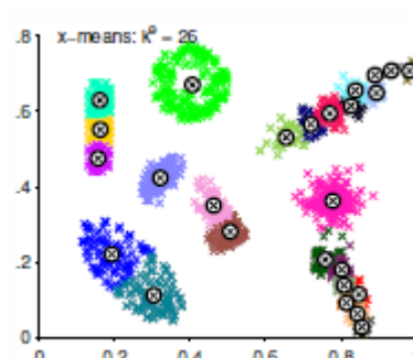
Σχήμα 3.4.8 Μονοτροπικές X-Means
