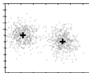
Σχήμα 3.3.2 Διαχωρισμός G-Means 2
