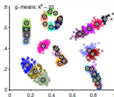
Σχήμα 3.4.9 Μονοτροπικές G-Means
